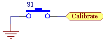
Gambar 4 Rangkaian Tactile Switch untuk Proses Calibrate
