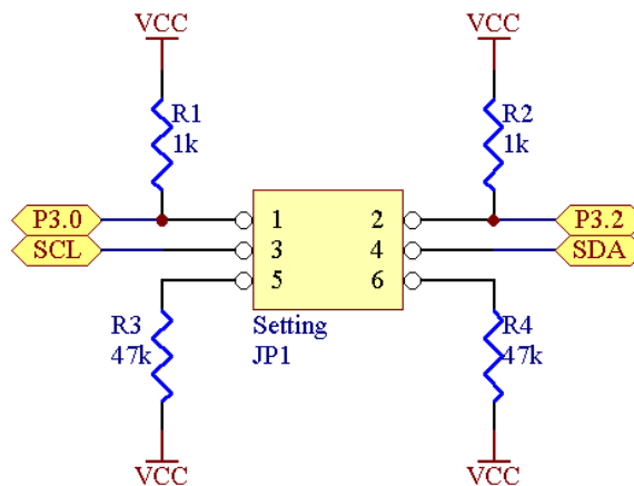
Gambar 3 Rangkaian Jumper untuk Pemilihan Resistor Pullup pada Jalur SCL & SDA
