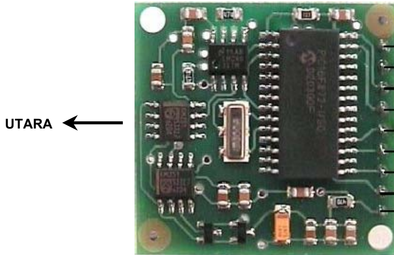
Gambar 5 Orientasi CMPS03 Robot Compass Module yang Menghasilkan Pembacaan 0°
