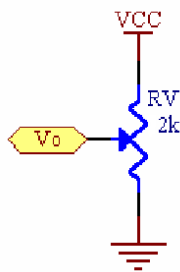
Gambar 2 Rangkaian Kontras untuk LCD Karakter 8x2
